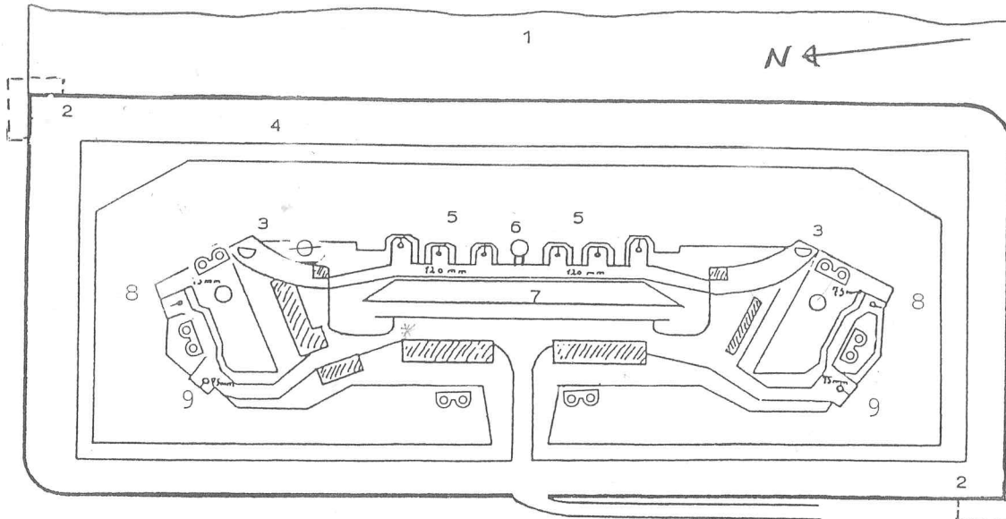
Fig. 6. Mosede Fort. Anlæg og armering.
